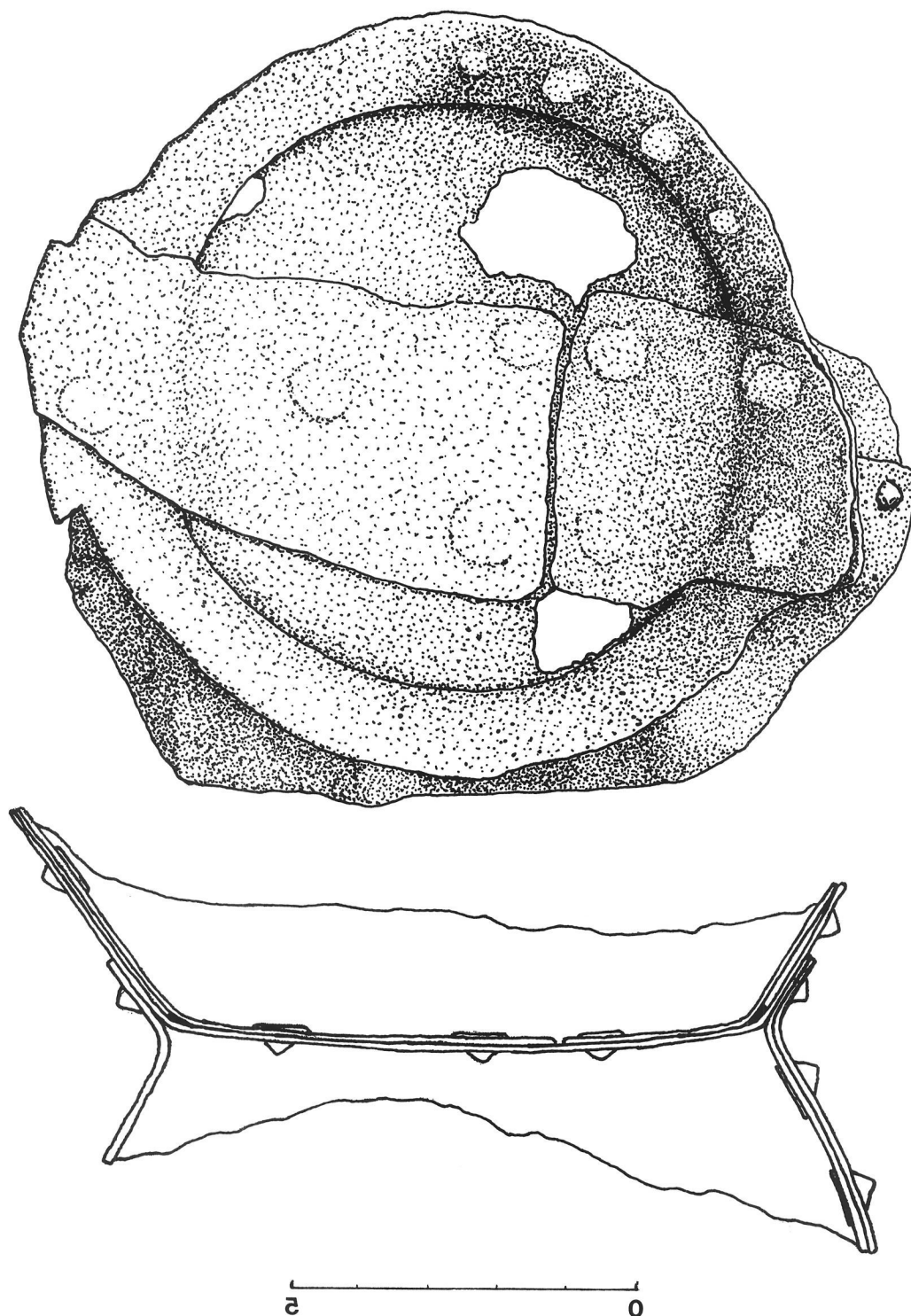
Figura 8. Fragmento de recipiente metálico.
