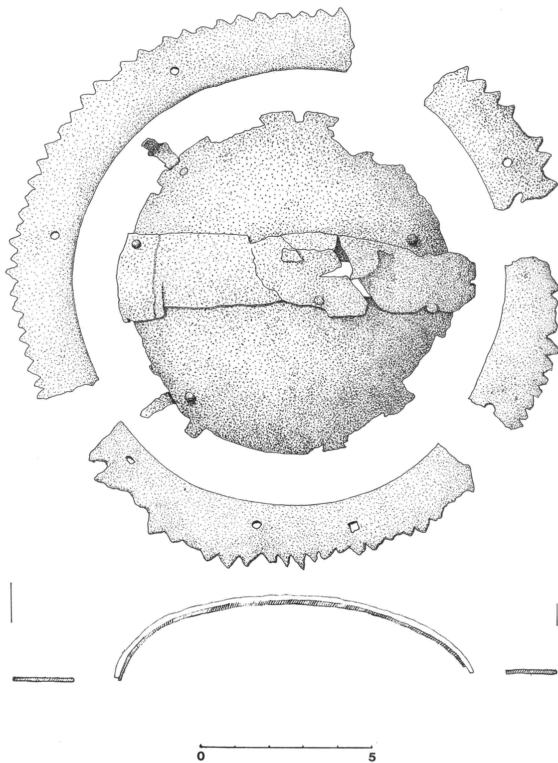
Figura 9. Umbo de escudo.
