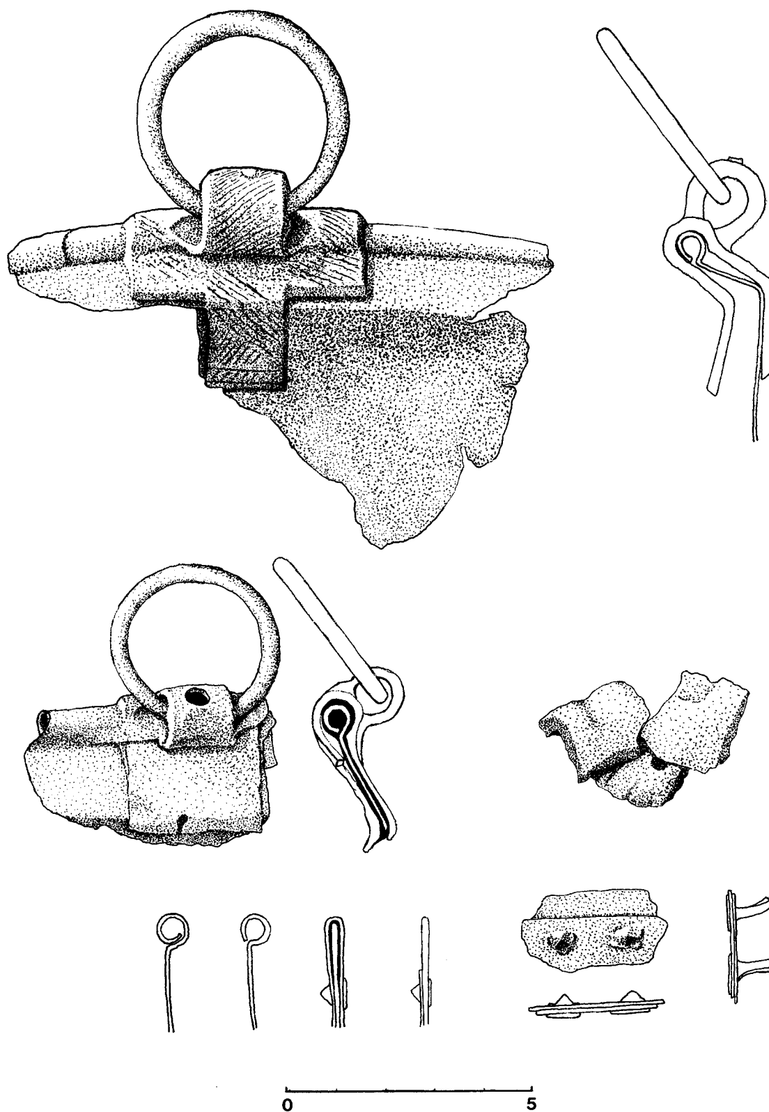
Figura 7. Fragmentos de calderos de tipo atlántico.
