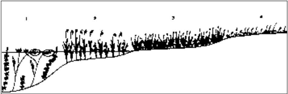
FIGURA 2. Transecto en la zona de los Ullals de Panxa. 1. Potamo-Vallisnerietum subas. nymphaeetosum albae . 2. Soncho-Cladietum marisci . 3. Comunidad de Phalaris arundinacea . 4. Orchido palustris-Centaureetum dracunculifoliae .
