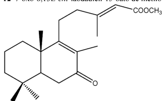
12 7-oxo-8,13E- ent -labdadien-15-oato de metilo
